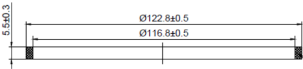
JUNTA CORRECTA
